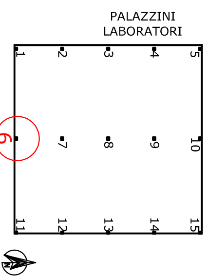
PIANTA PILASTRI
